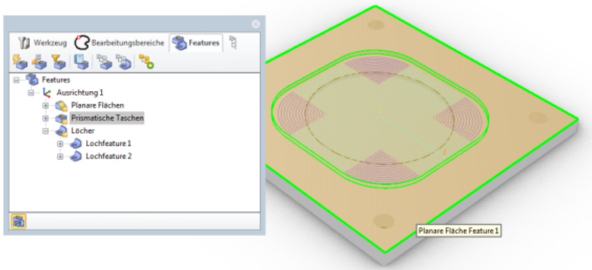
Anzeige von Features – Hier: Prismatische Taschen
